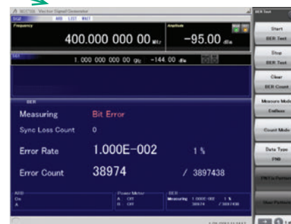
BER Function
